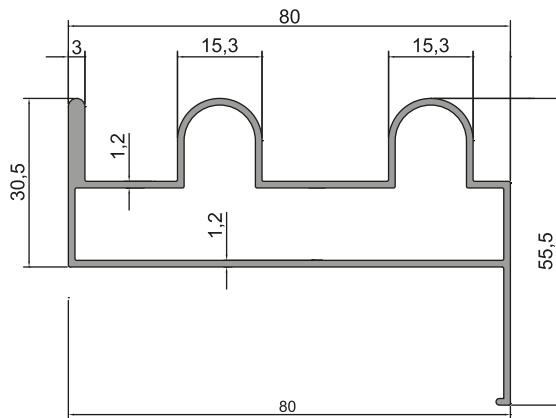
14-030 (0,967 kg/m)
