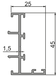
14-004 (0,439 kg/m)
