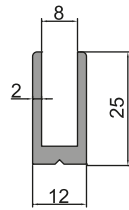
14-023 (0,354 kg/m)
