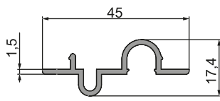
14-007 (0,306 kg/m)
