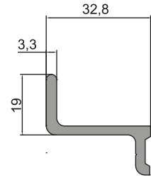
14-026 (0,507 kg/m)
