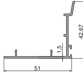
14-005 (0,447 kg/m)
