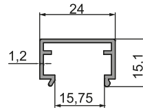
14-009 (0,206 kg/m)
