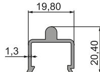
14-008 (0,242 kg/m)
