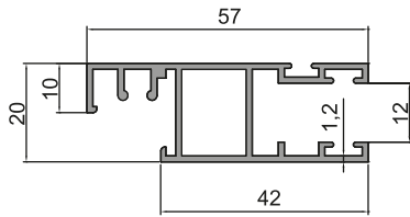
14-027 (0,607 kg/m)
