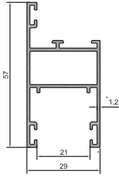
14-014 (0,616 kg/m)
