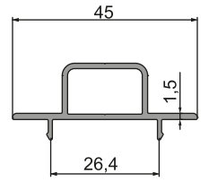
14-006 (0,343 kg/m)
