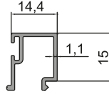
14-024 (0,177 kg/m)
