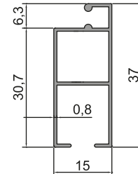
14-031 (0,243 kg/m)
