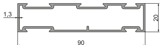
14-012 (0,927 kg/m)
