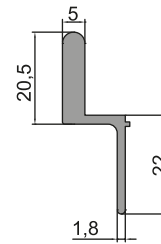
14-025 (0,421 kg/m)
