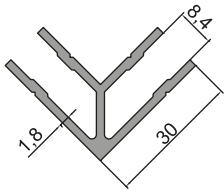
14-022 (0,553 kg/m)
