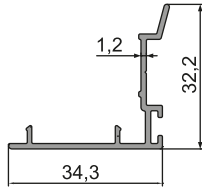
14-018 (0,268 kg/m)
