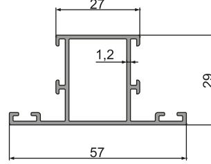
14-015 (0,550 kg/m)
