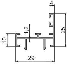
14-017 (0,322 kg/m)
