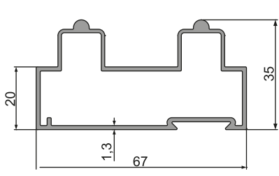
14-013 (0,822 kg/m)
