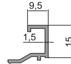
14-029 (0,178 kg/m)
