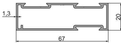
14-011 (0,692 kg/m)
