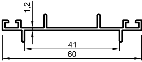
No : 5309 Düşey-Yatay Alt Profili 0,320 kg/m
