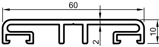
No : 4194 Kapak Profili 0,600 kg/m
