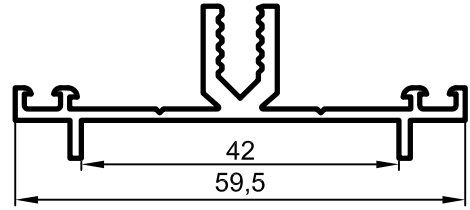
No : 3689 Düşey-Yatay Alt Profili 0,530 kg/m
