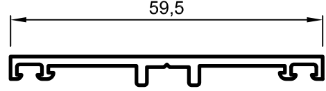
No : 3688 Kapak Profili 0,375 kg/m
