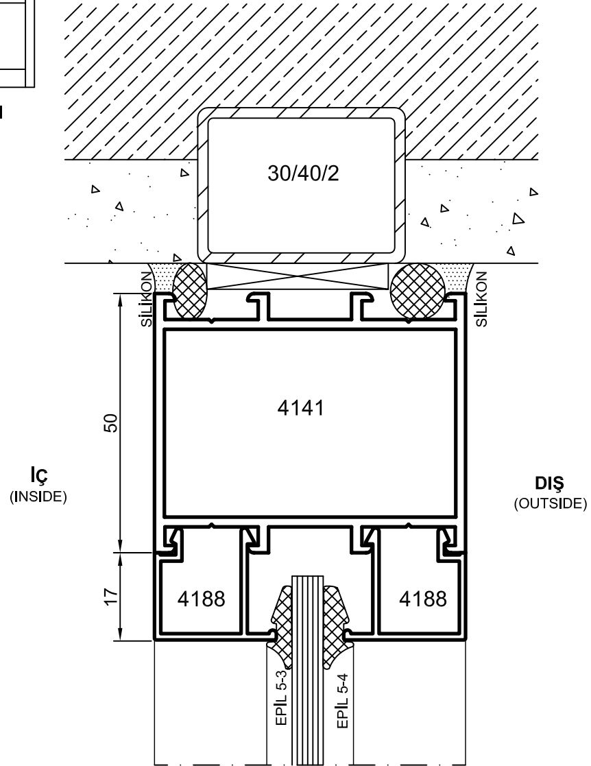
VİTRİN DOĞRAMASI
