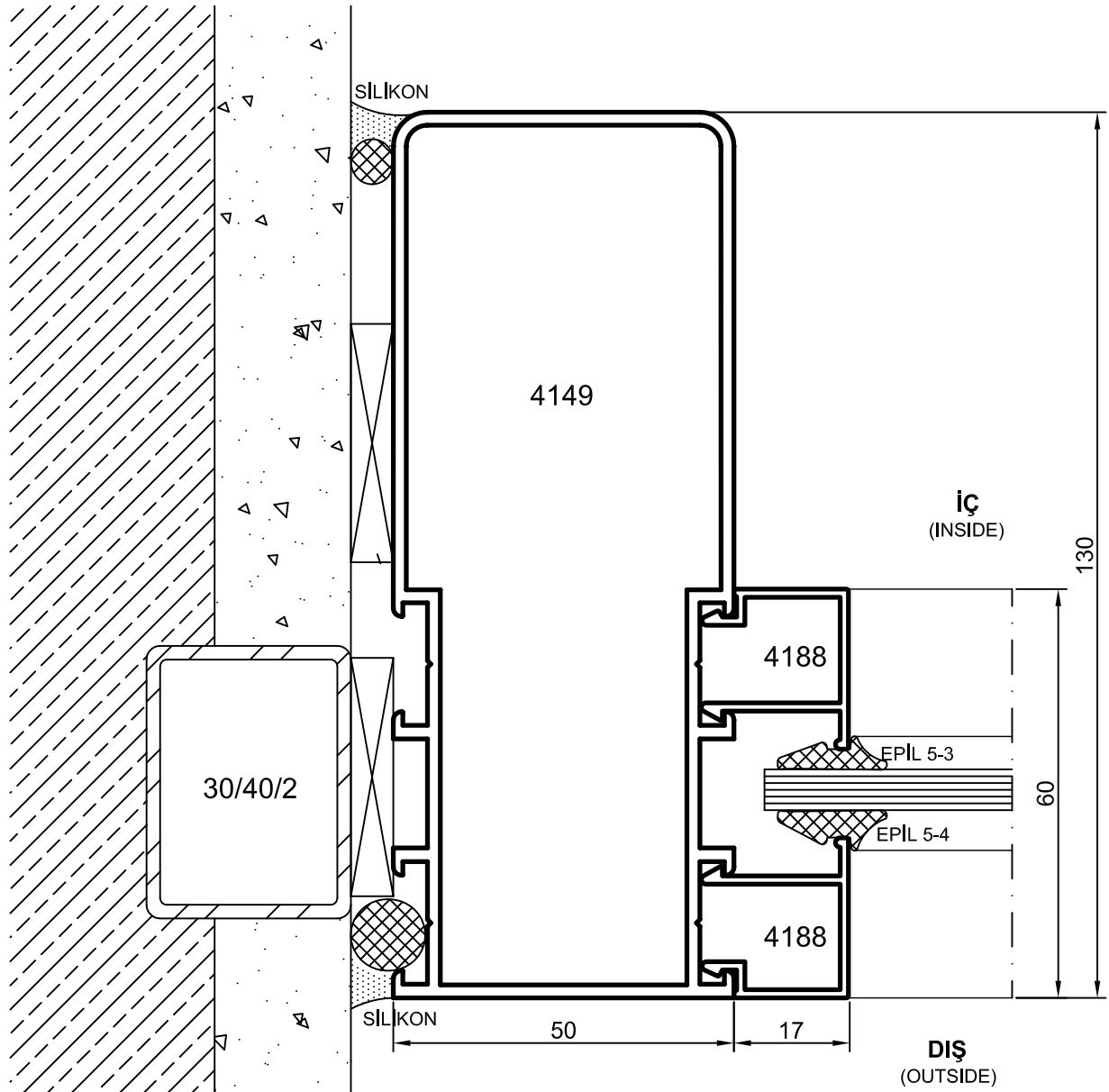
VİTRİN DOĞRAMASI
