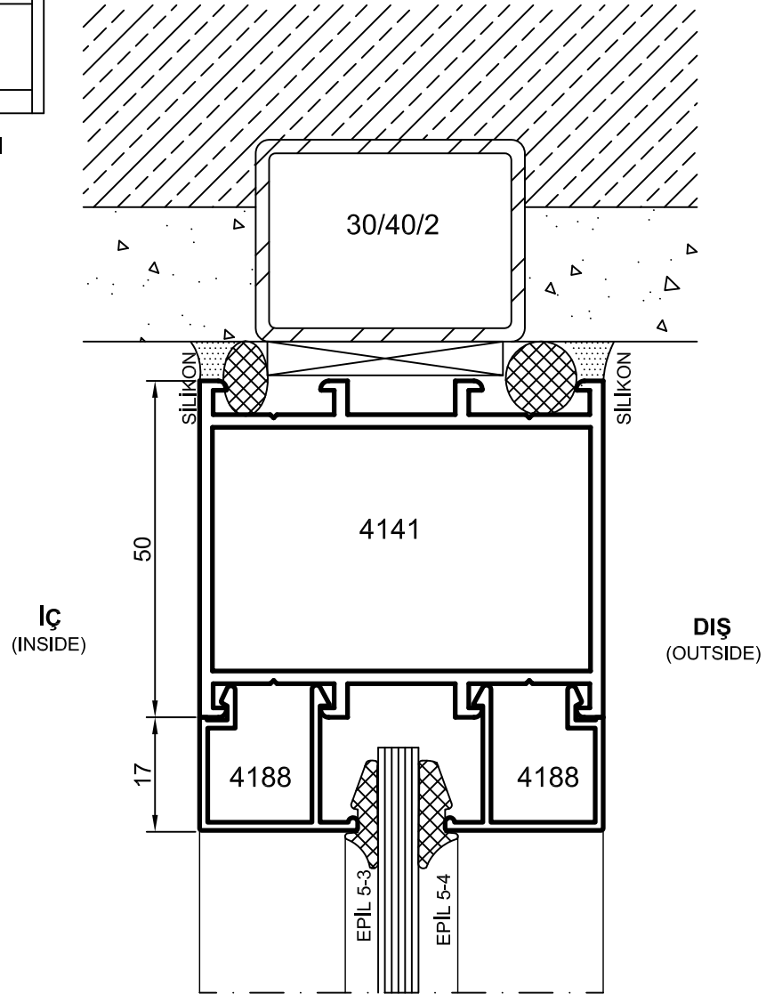
VİTRİN DOĞRAMASI
