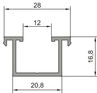
TEK CAM ÇITA PROFİLİ 26-018 (0,270kg/m)
