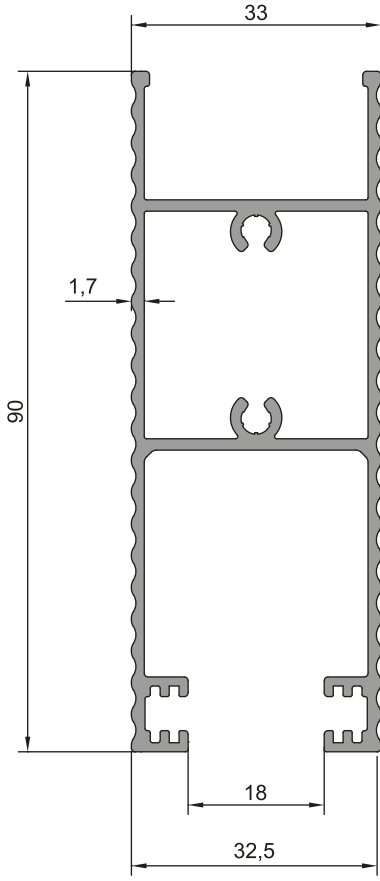
DEKORATİF ETEK PROFİLİ 26-013 (1,167kg/m) Jx: 7,57 cm 4 / Jy: 29,90 cm 4
