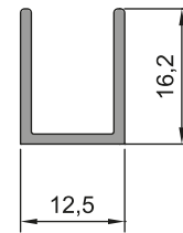
U PROFİLİ 05-001 (0,146kg/m)
