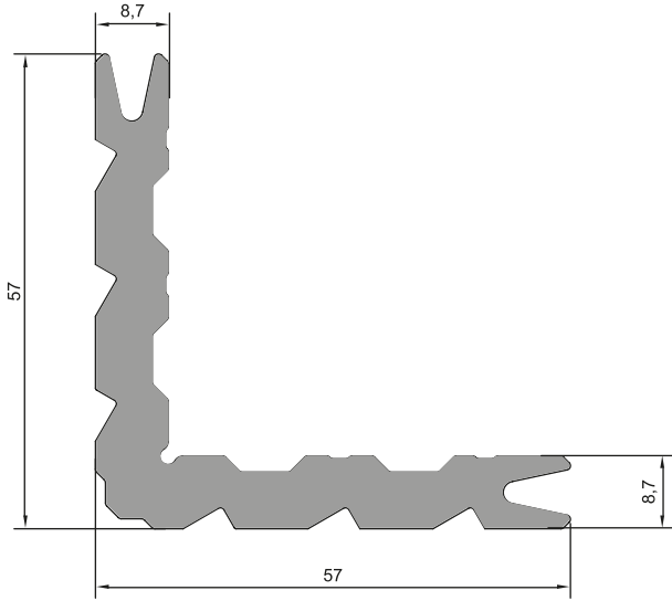
KÖŞE TAKOZU 22-065 (1,958kg/m)
