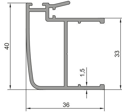
ORTA KANAT PROFİLİ 26-008 (0,648kg/m) Jx: 5,07 cm 4 / Jy: 2,35 cm 4
