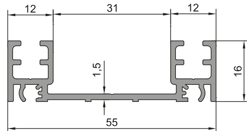
KASA PROFİLİ 26-004 (0,565 kg/m) Jx: 8,10 cm 4 / Jy: 0,49 cm 4
