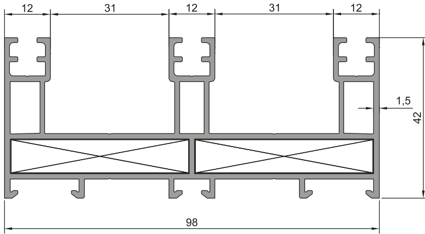
3'LÜ KASA PROFİLİ 26-003 (1,763 kg/m) Jx: 70,31 cm 4 / Jy: 9,77 cm 4
