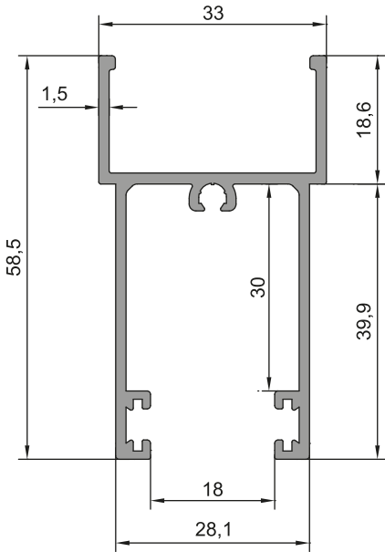
ETEK PROFİLİ 26-011 (0,735kg/m) Jx: 4,32 cm 4 / Jy: 7,83 cm 4
