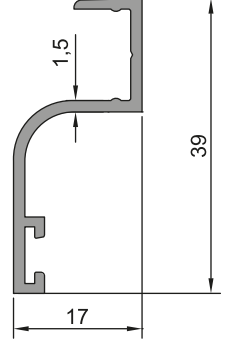
DAMLALIK PROFİLİ 26-015 (0,267kg/m)
