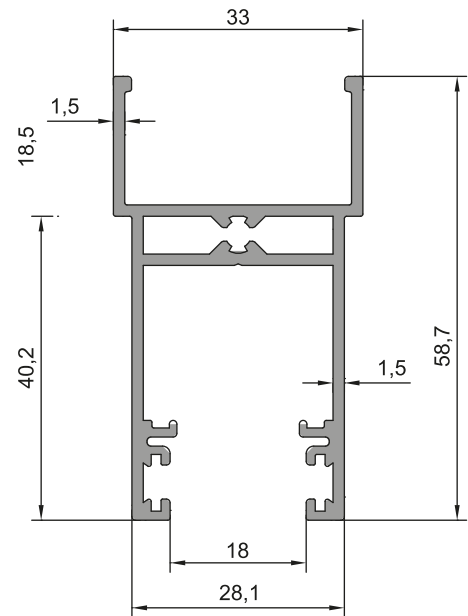
ETEK PROFİLİ 26-012 (0,864kg/m) Jx: 4,65 cm 4 / Jy: 8,40 cm 4
