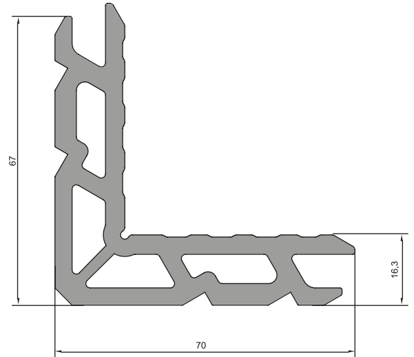
KÖŞE TAKOZU 21-047 (3,220kg/m)
