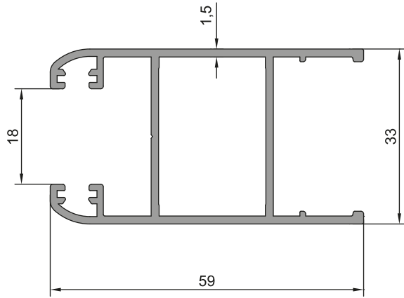
KANAT PROFİLİ 26-007 (0,822kg/m) Jx: 5,55 cm 4 / Jy: 8,44 cm 4
