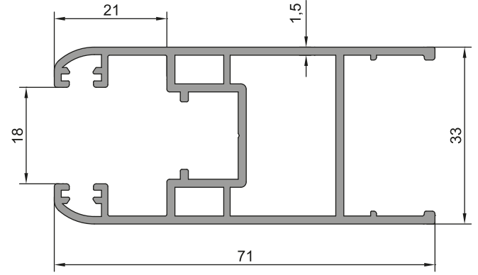
PVC İSP. KANALLI KANAT PROFİLİ 26-006 (1,090kg/m) Jx: 7,01 cm 4 / Jy: 14,70 cm 4
