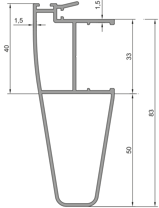
TAKVİYELİ ORTA KANAT PROFİLİ 26-010 (1,085kg/m) Jx: 31,47 cm 4 / Jy: 4,61 cm 4
