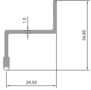
SİNEKLİK RAY PROFİLİ 16-010 (0,261kg/m)
