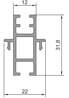
DÖRTLÜ KANAT ADAPTÖRÜ 26-017 (0,413kg/m)
