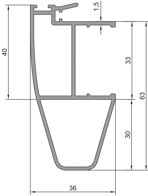
TAKVİYELİ ORTA KANAT PROFİLİ 26-009 (0,934kg/m) Jx: 16,60 cm 4 / Jy: 3,64 cm 4
