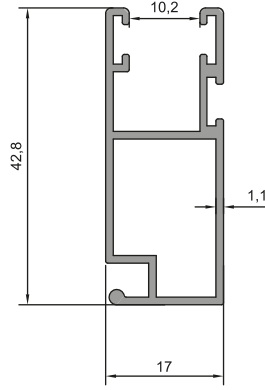
SİNEKLİK KANAT PROFİLİ 16-005 (0,419kg/m)
