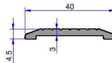
4201 0.312 kg/m
