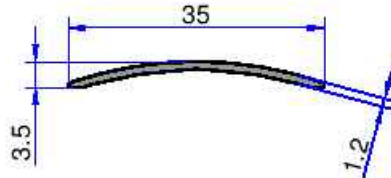
5400 0.106 kg/m
