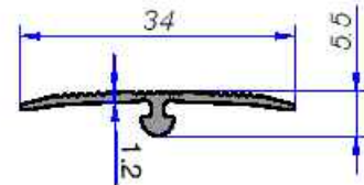
10-2723 0.127 kg/m
