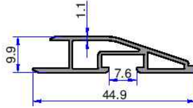
10987 0.313 kg/m
