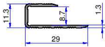
10-2707 0.161 kg/m
