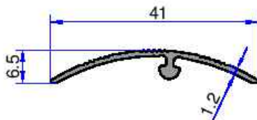
10-2722 0.157 kg/m
