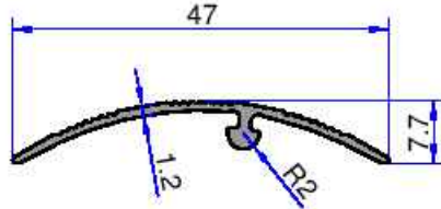
10-2721 0.176 kg/m
