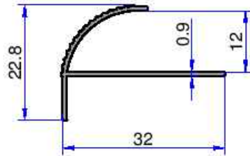
6126 0.160 kg/m
