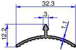
5305 0.137 kg/m
