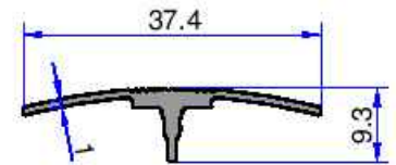
6124 0.168 kg/m
