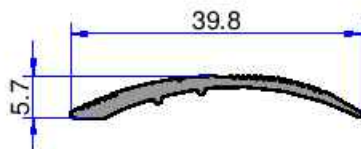
10167 0.190 kg/m
