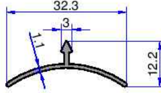
5306 0.127 kg/m
