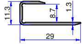
4712 0.160 kg/m
