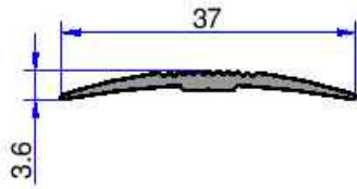
6505 0.147 kg/m
