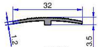
5089 0.128 kg/m
