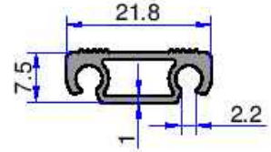
5379 0.190 kg/m
