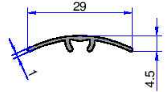
5381 0.107 kg/m
