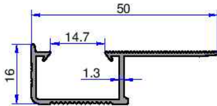
5169 0.279 kg/m
