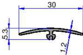
4999 0.116 kg/m
