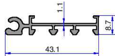
10920 0.312 kg/m
