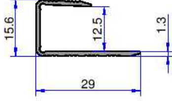
10-2726 0.177 kg/m
