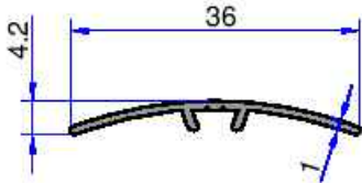
5191 0.117 kg/m
