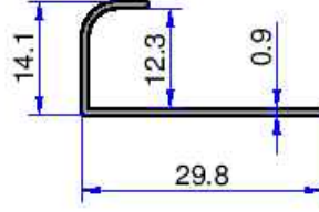
6125 0.118 kg/m
