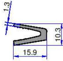
3876 0.169 kg/m
