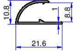
5320 0.115 kg/m
