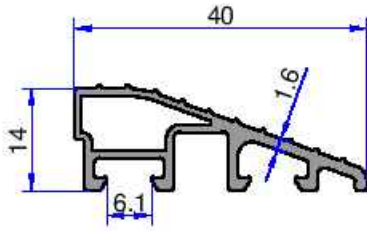
11050 0.351 kg/m
