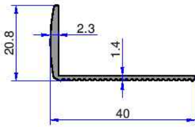
5268 0.224 kg/m
