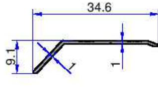
6324 0.097 kg/m
