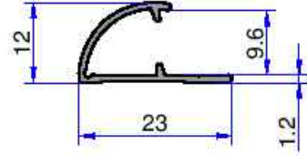
5595 0.122 kg/m
