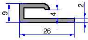
5559 0.244 kg/m
