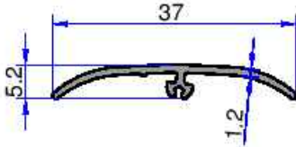
9929 0.147 kg/m
