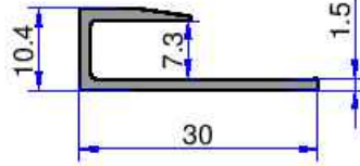
6428 0.201 kg/m
