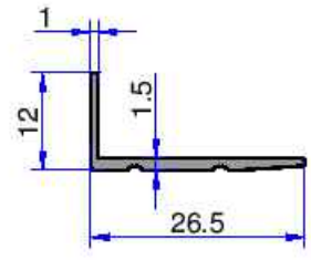
4996 0.126 kg/m
