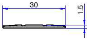
4998 0.106 kg/m
