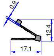
3852 0.089 kg/m
