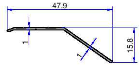
6323 0.137 kg/m
