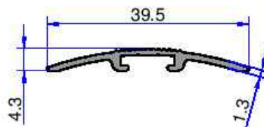
5104 0.160 kg/m
