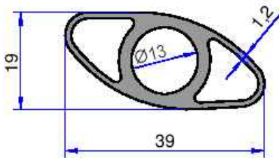
4518 0.595 kg/m
