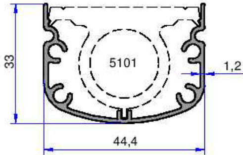
5100 0.458 kg/m
