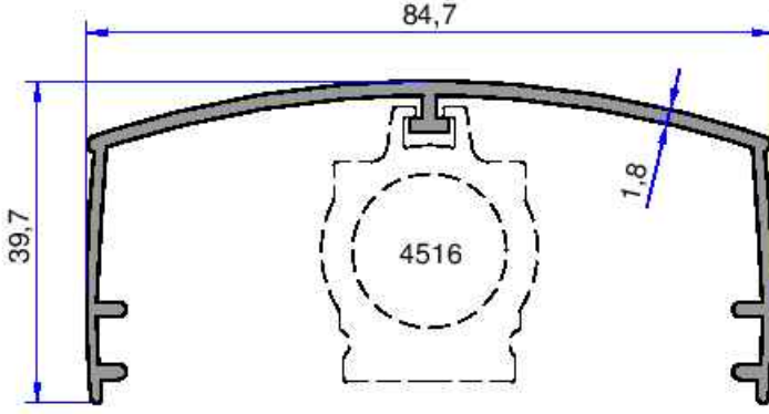
4517 0.757 kg/m
