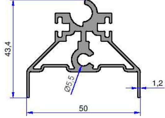
5251 1.011 kg/m
