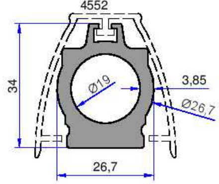
4516 1.093 kg/m
