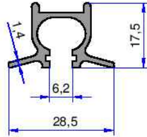
3187 0.315 kg/m
