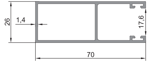
09-012 (0,777 kg/m)
