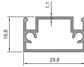
10 - 007 (0,346 kg/m)
