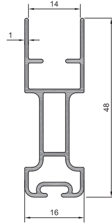
10 - 012 (0,415 kg/m)
