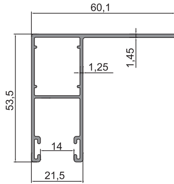
09-002 (0,702 kg/m)
