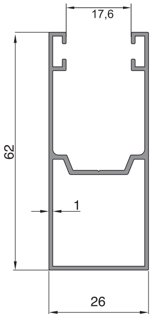
09-4730 (0,553 kg/m)
