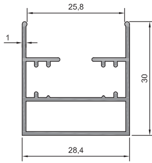
10 - 013 (0,379 kg/m)
