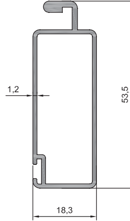
10 - 010 (0,495 kg/m)
