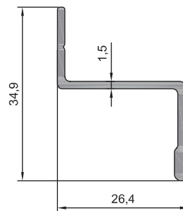
16 - 010 (0 261 kg/m)
