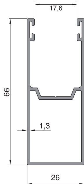
09-4729 (0,698 kg/m)
