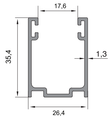
09-026 (0,455 kg/m)
