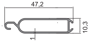
09-006 (0,286 kg/m)
