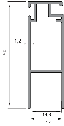
10 - 025 (0,469 kg/m)
