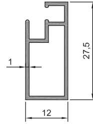
10 - 005 (0,220 kg/m)
