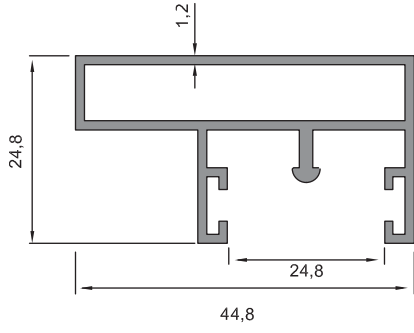
15 - 004 (0,531 kg/m)
