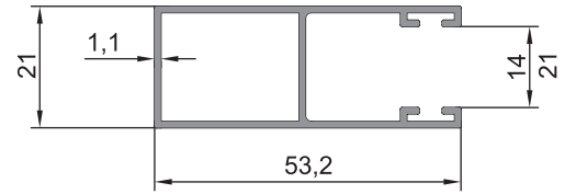
09-014 (0,484 kg/m)
