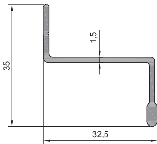
16 - 009 (0,287 kg/m)
