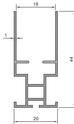
10 - 015 (0,388 kg/m)
