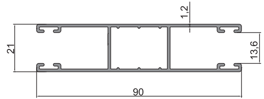
09-003 (0,828 kg/m)
