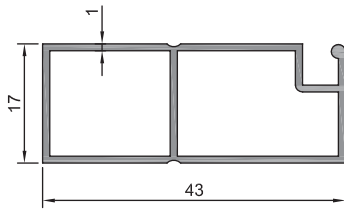
10 - 006 (0,370 kg/m)
