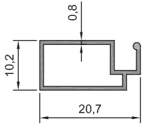
10 - 001 (0,135 kg/m)
