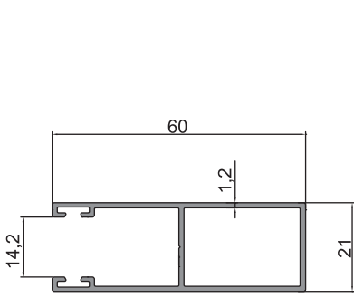
09-001 (0,557 kg/m)
