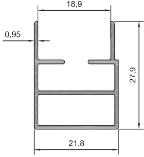
10 - 011 (0,282 kg/m)
