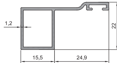
10 - 009 (0,321 kg/m)
