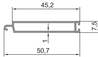
09-016 (0,302 kg/m)
