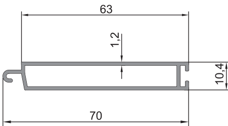
09-015 (0,508 kg/m)
