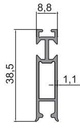
09-008 (0,319 kg/m)
