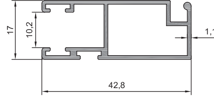
16 - 005 (0,419 kg/m)
