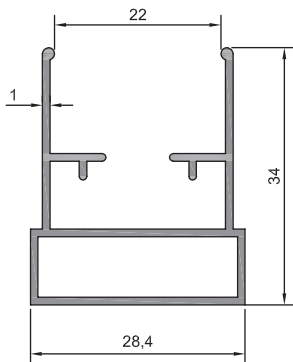
10 - 014 (0,382 kg/m)
