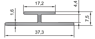
07 - 004 (0,252 kg/m)
