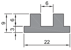
06 - 003 (0,342 kg/m)
